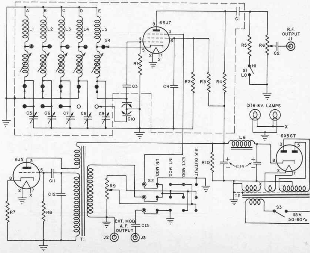
Fig. 1 Wiring Diagram, 3432
